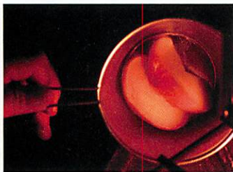
スノーピークス社製の焚き火台と、リング1個が収まる大きさの同社製ダッチオーブン「コロダッチ」で焼きリングをつくる。食べやすい大きさにクシ切りしたリングを、焦げないようにアルミホイルで包み、まず2〜3分強火にした後、弱火で12〜15分火にかける
